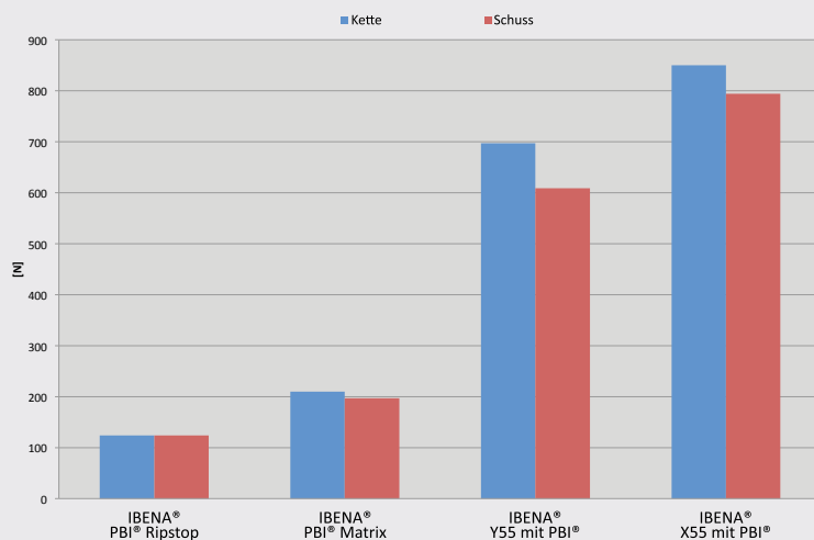
Durchschnittliche Weiterreißfestigkeit gemäß DIN EN ISO 13937-2, Anhang D
