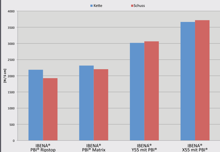
Durchschnittliche Zugfestigkeit gemäß DIN EN ISO 13934-1
