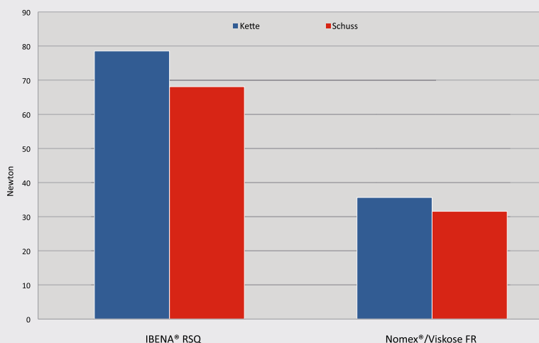
Durchschnittliche Weiterreißfestigkeit gemäß DIN EN ISO 13937-2
