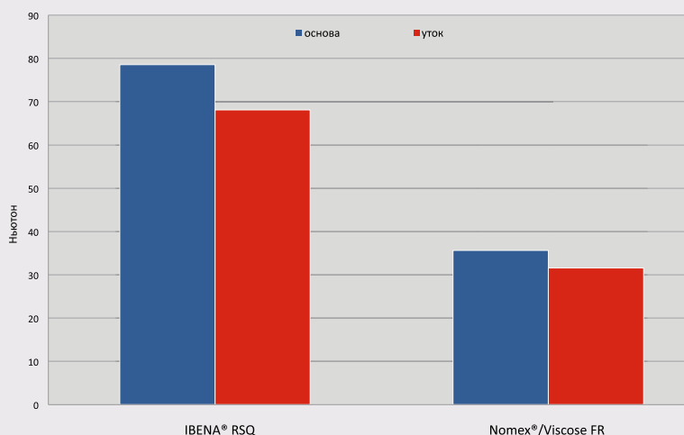
Средняя раздирающая нагрузка согласно EN ISO 13937-2
