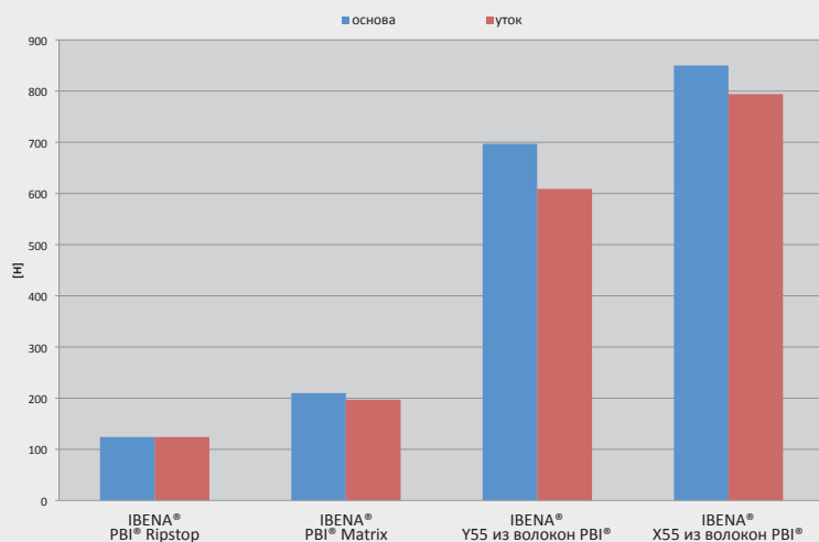
Средние показатели раздирающей нагрузки согласно DIN EN ISO 13937-2
