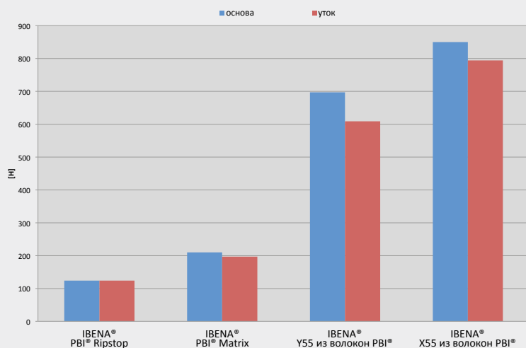
Средние показатели раздирающей нагрузки согласно DIN EN ISO 13937-2 (D)
