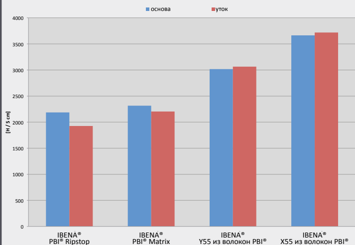
Средние показатели разрывной нагрузки согласно DIN EN ISO 13934-1
